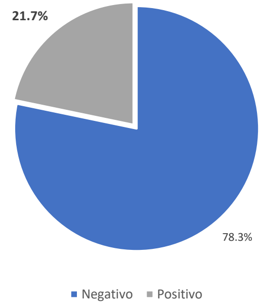
Positividade CEASA
