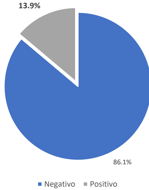
Positividade Geral
